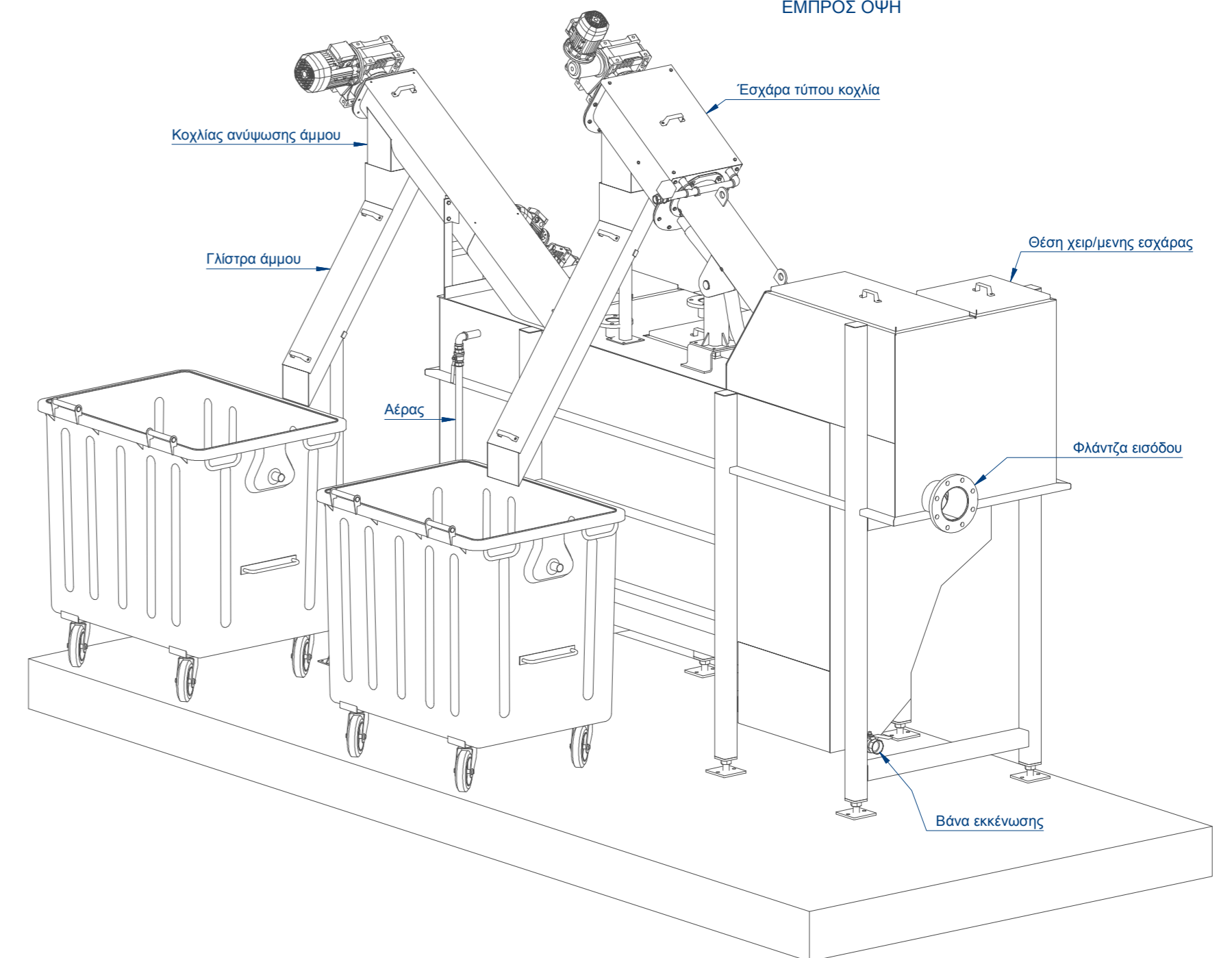
ΟΨΗ ΤΡΙΩΝ ΔΙΑΣΤΑΣΕΩΝ
