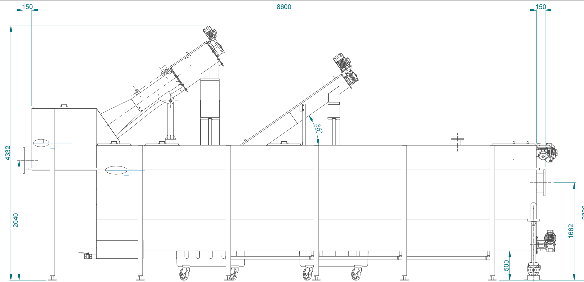
ΠΛΑΓΙΑ ΟΨΗ
