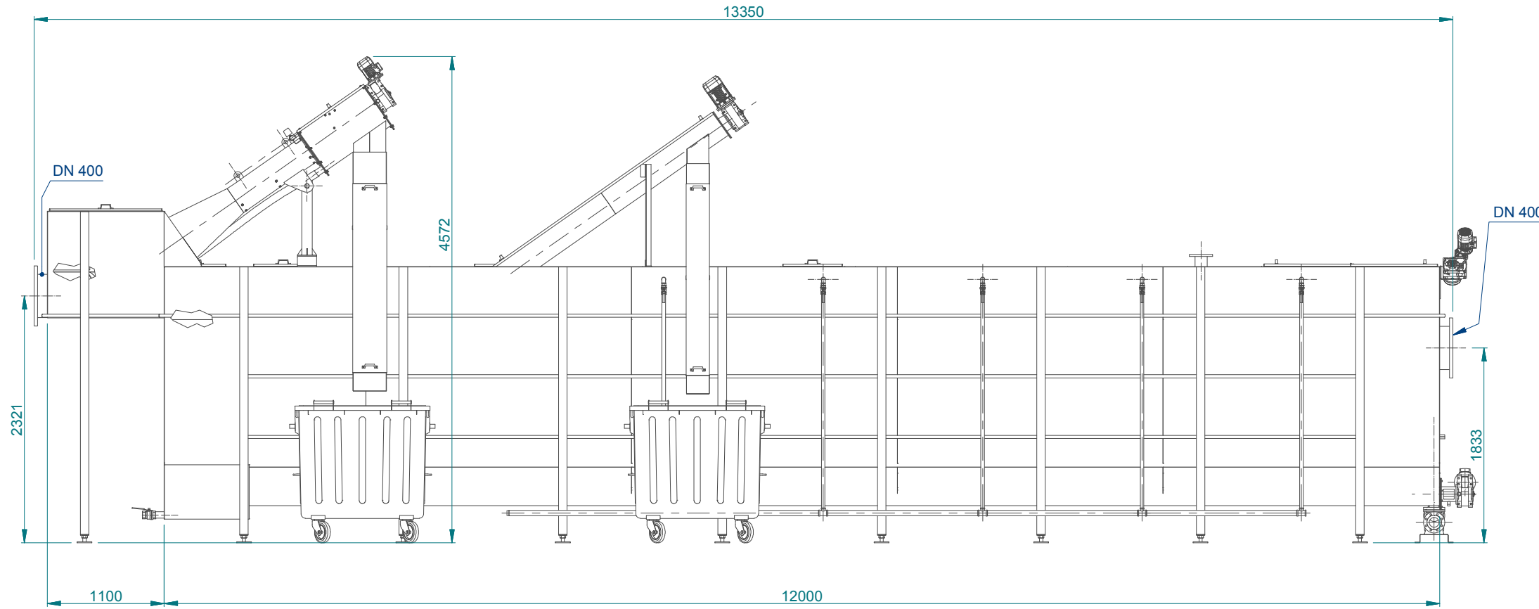
ΠΛΑΓΙΑ ΟΨΗ
