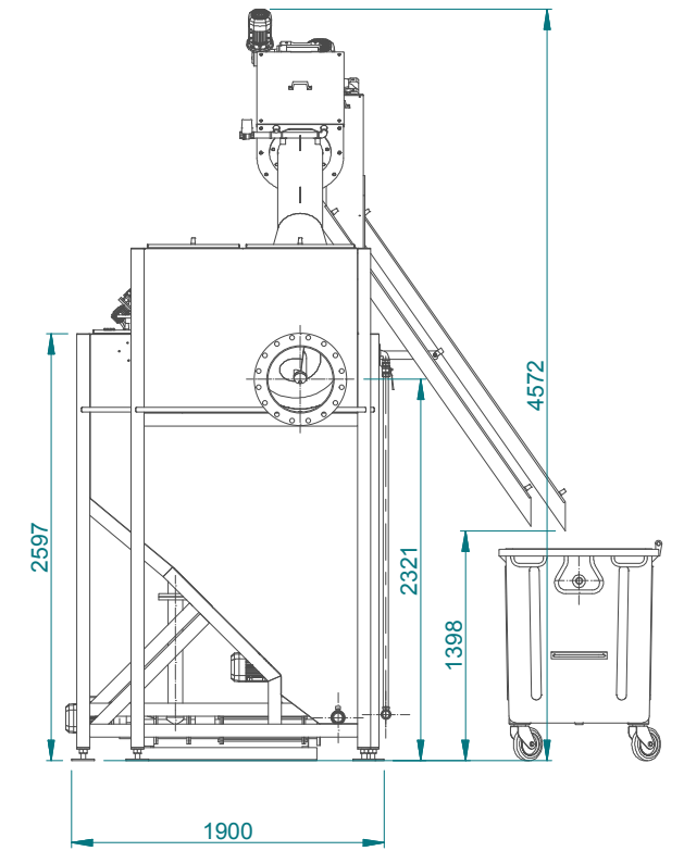
ΕΜΠΡΟΣ & ΟΨΗ
