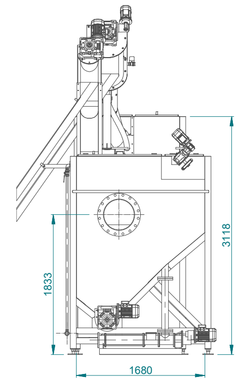
ΠΙΣΩ ΟΨΗ
