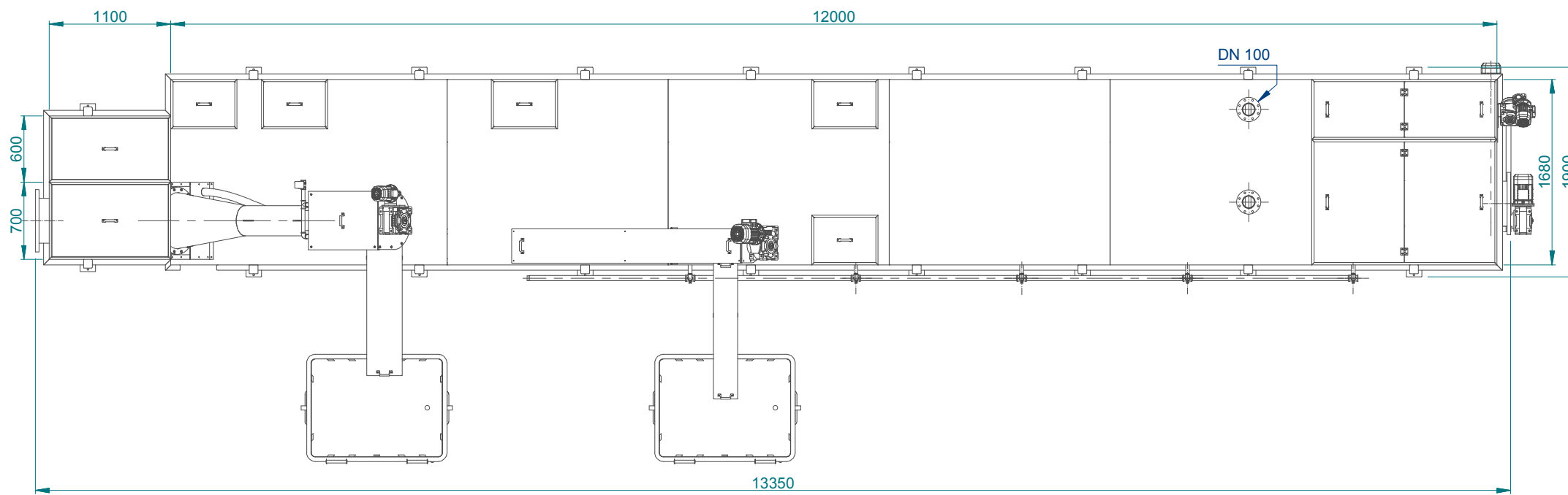
ΑΝΩ ΟΨΗ
