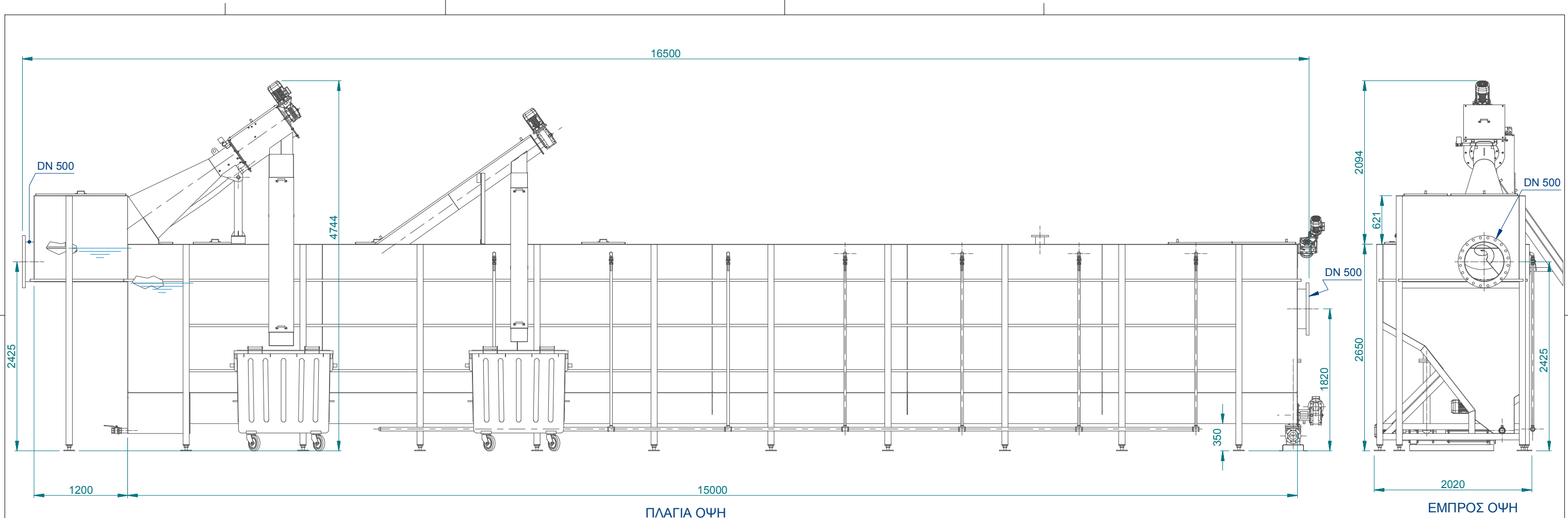
ΠΛΑΓΙΑ ΟΨΗ
